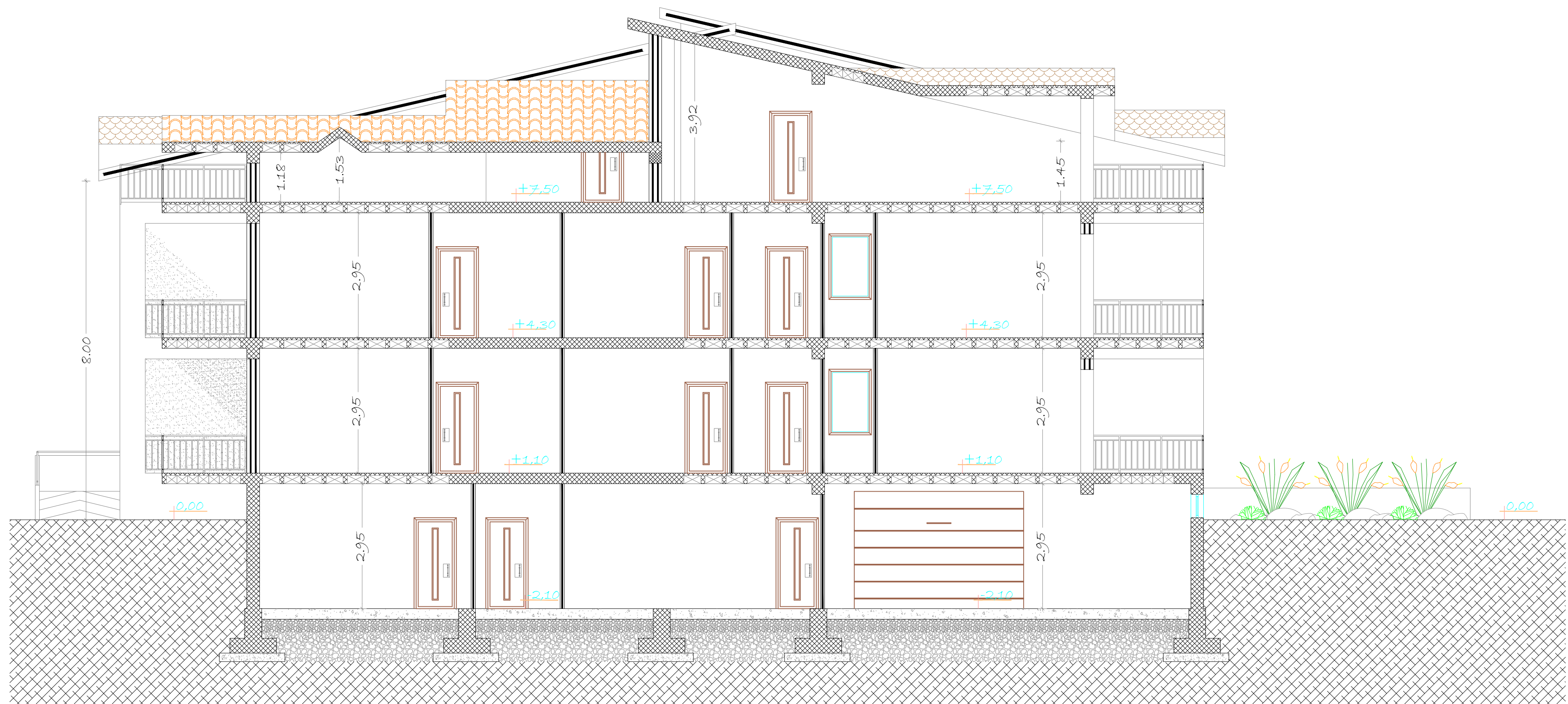
SEZIONE D-D rapp. 1:100
