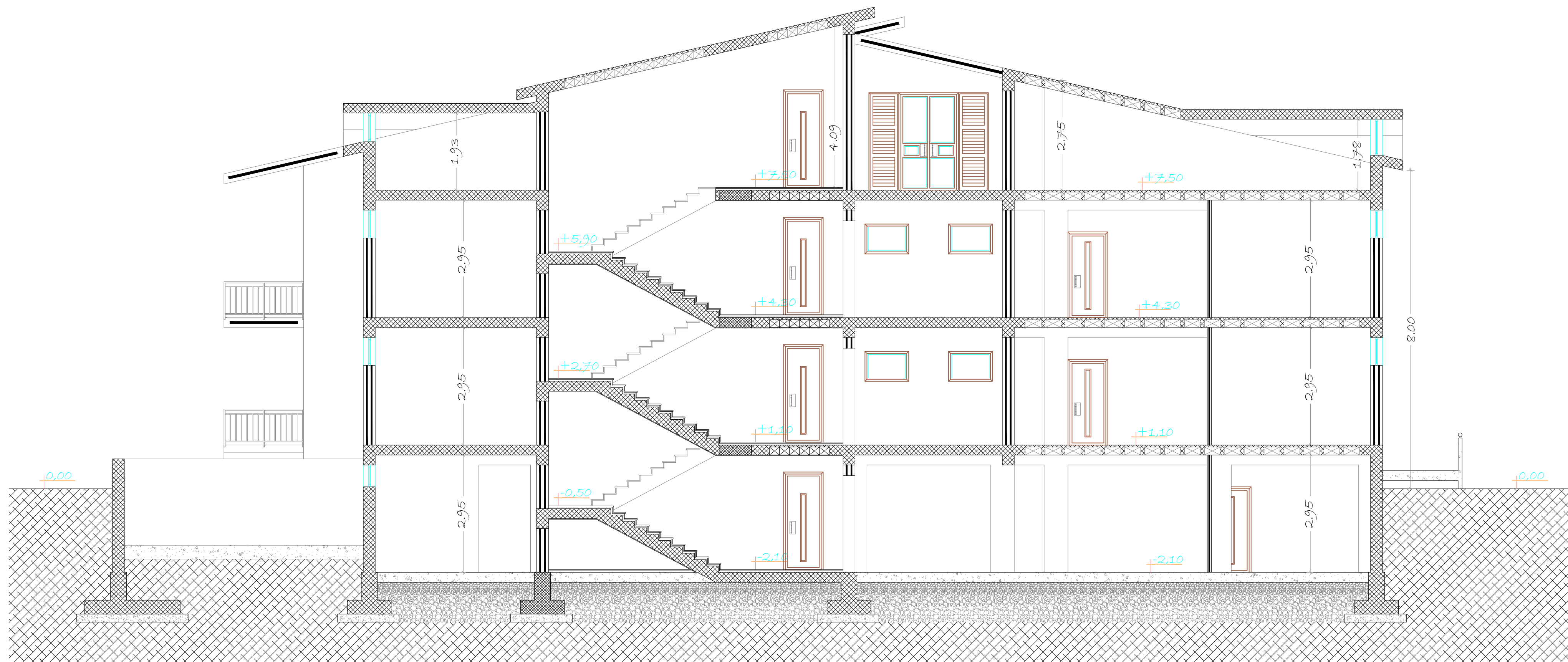
SEZIONE C-C rapp. 1:100
