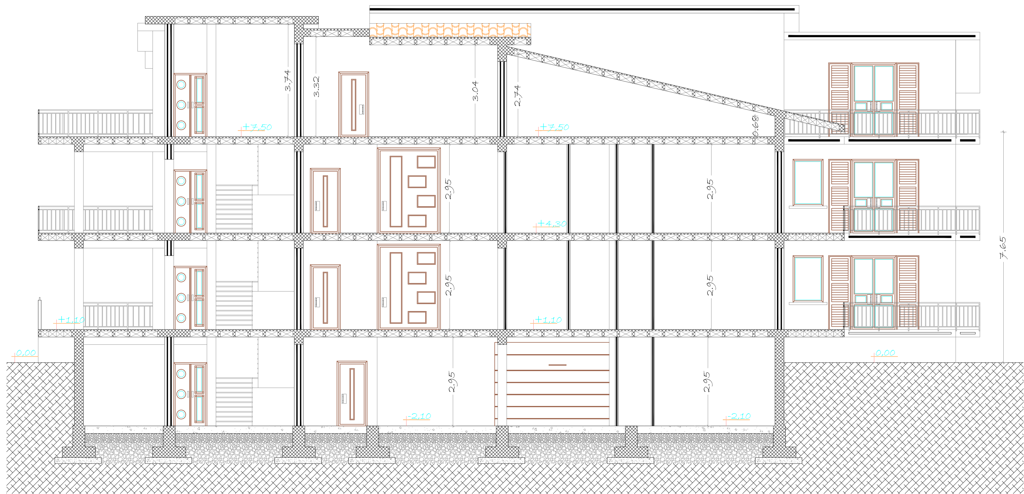
SEZIONE A-A rapp. 1:100
