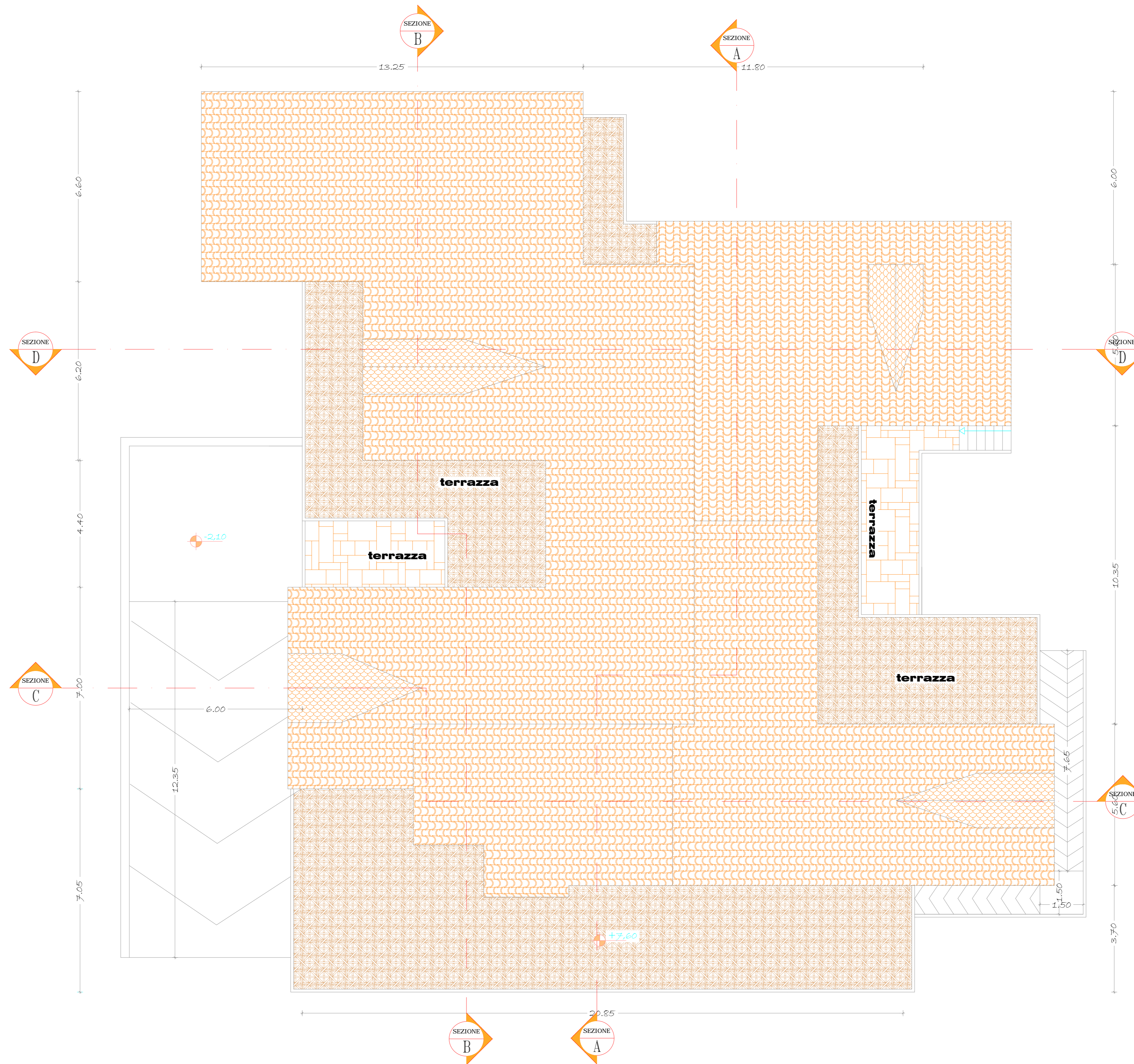
PIANTA DELLE COPERTURE rapp. 1:100
