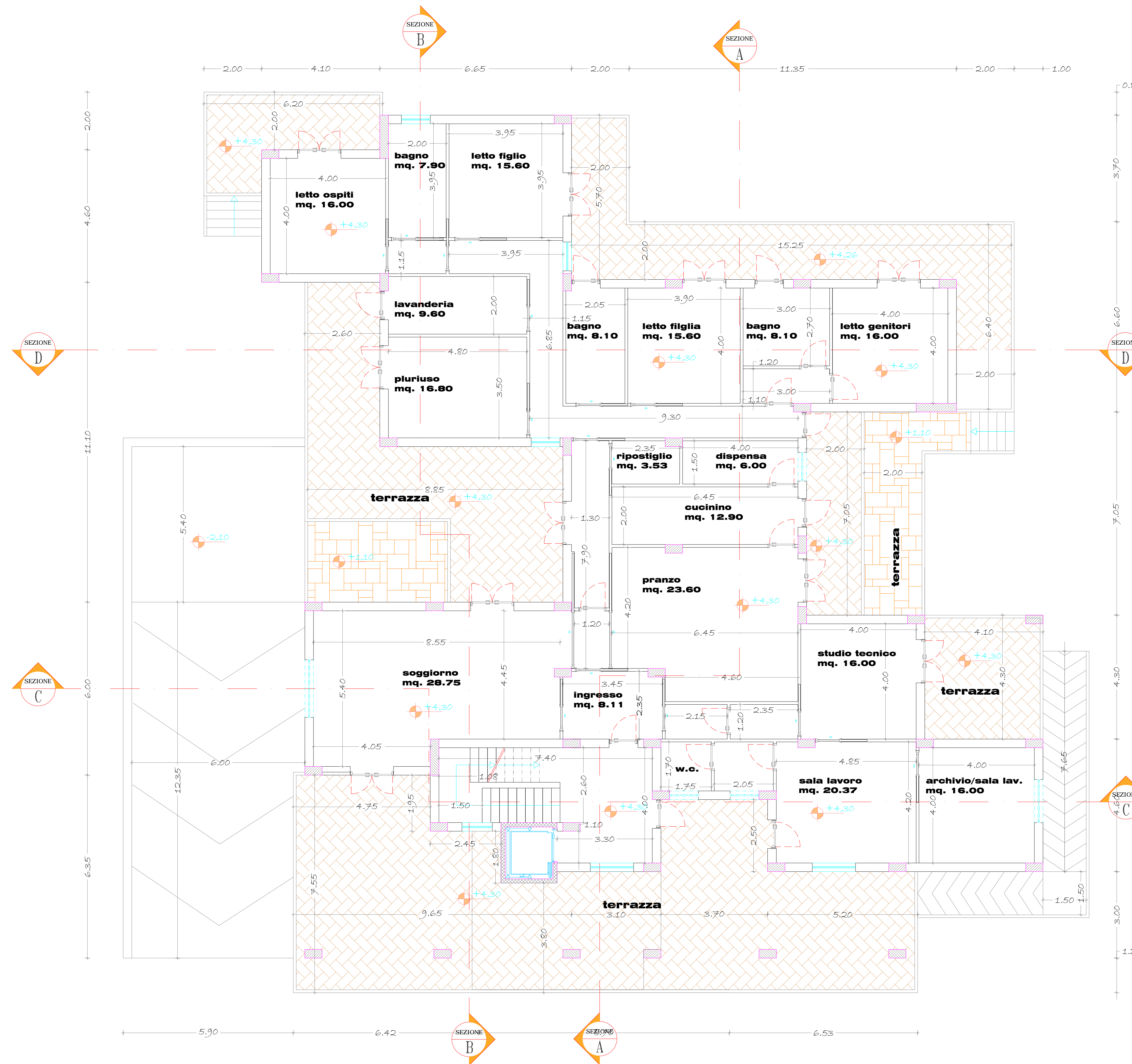
PIANTA PIANO PRIMO rapp. 1:100
