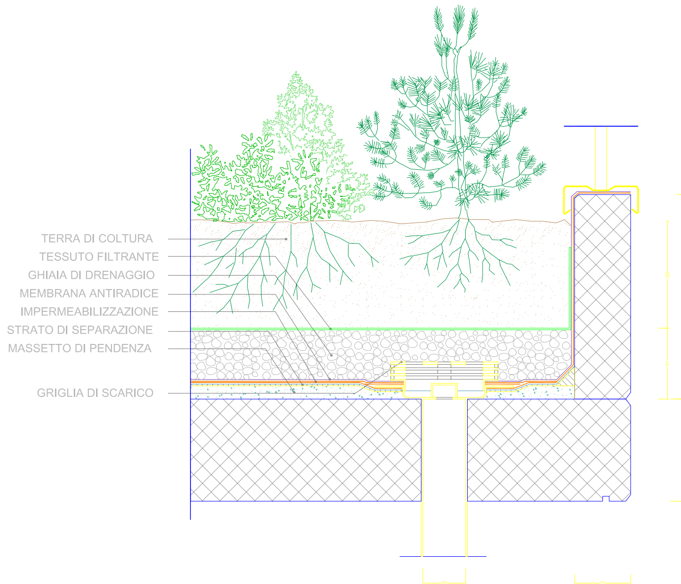
PARTICOLARE GIARDINO PENSILE scala 1:20
