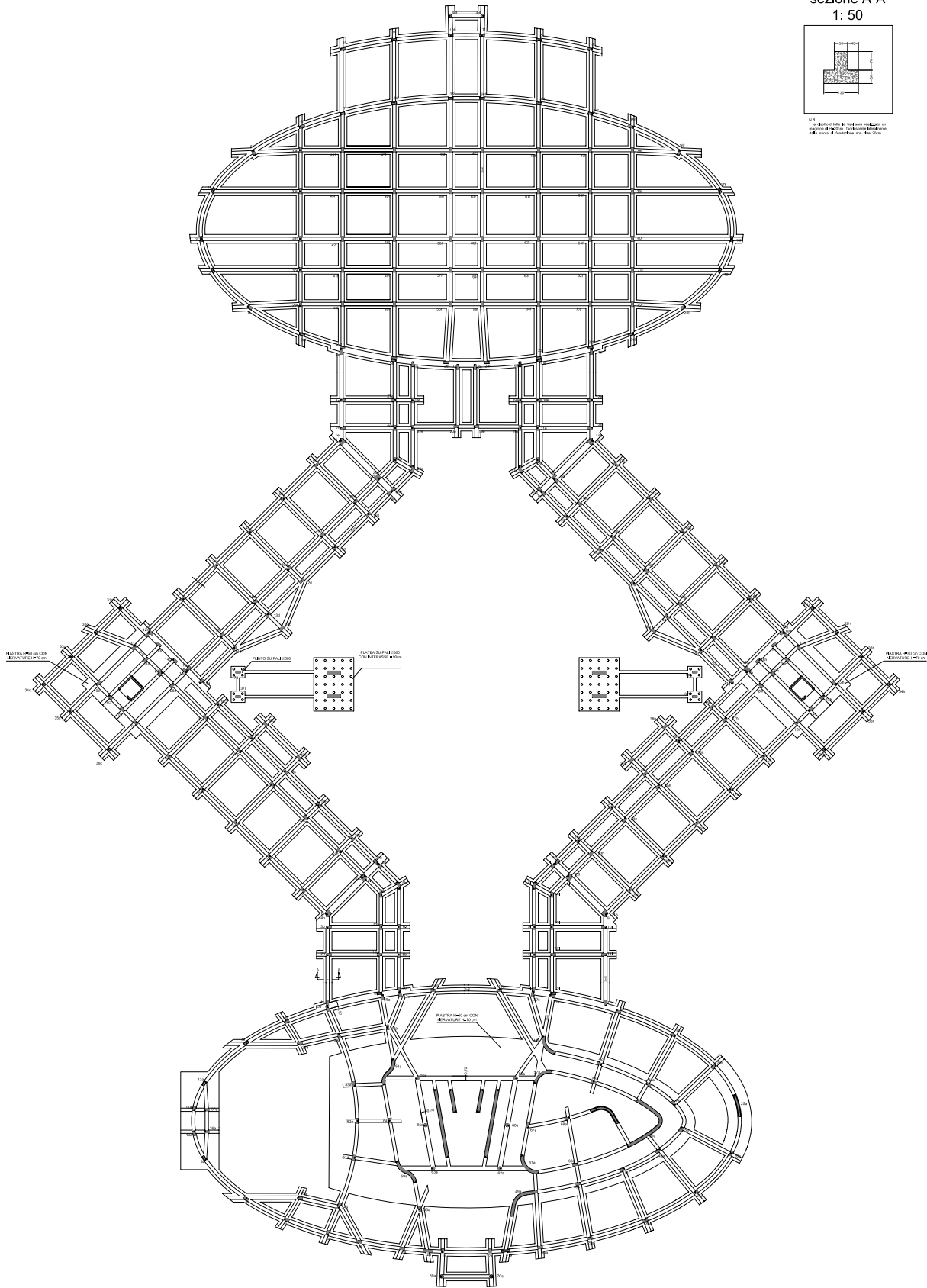
PIANTA DELLE FONDAZIONI scala 1:200
