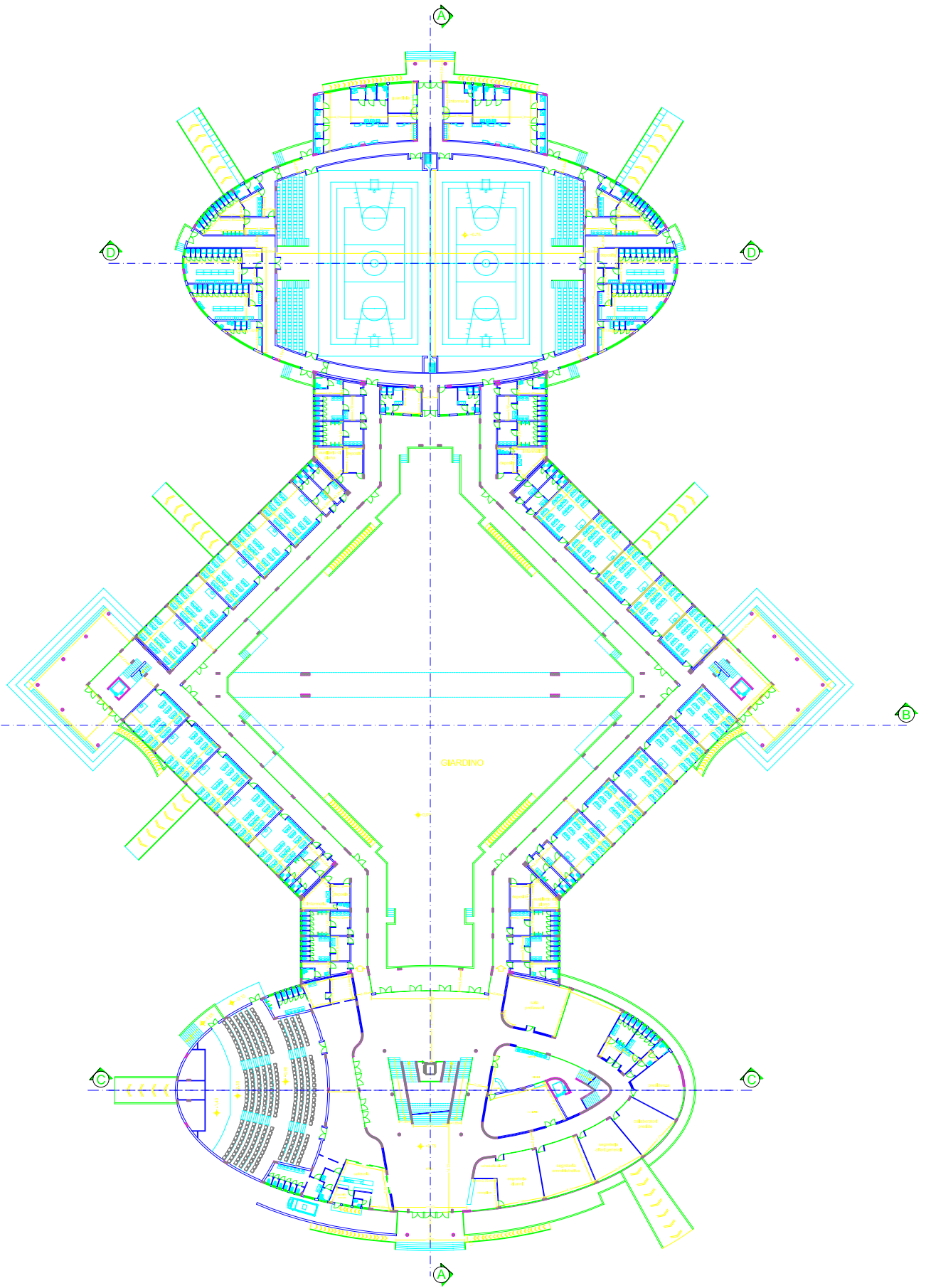
PIANTA PIANO RIALZATO scala 1:200
