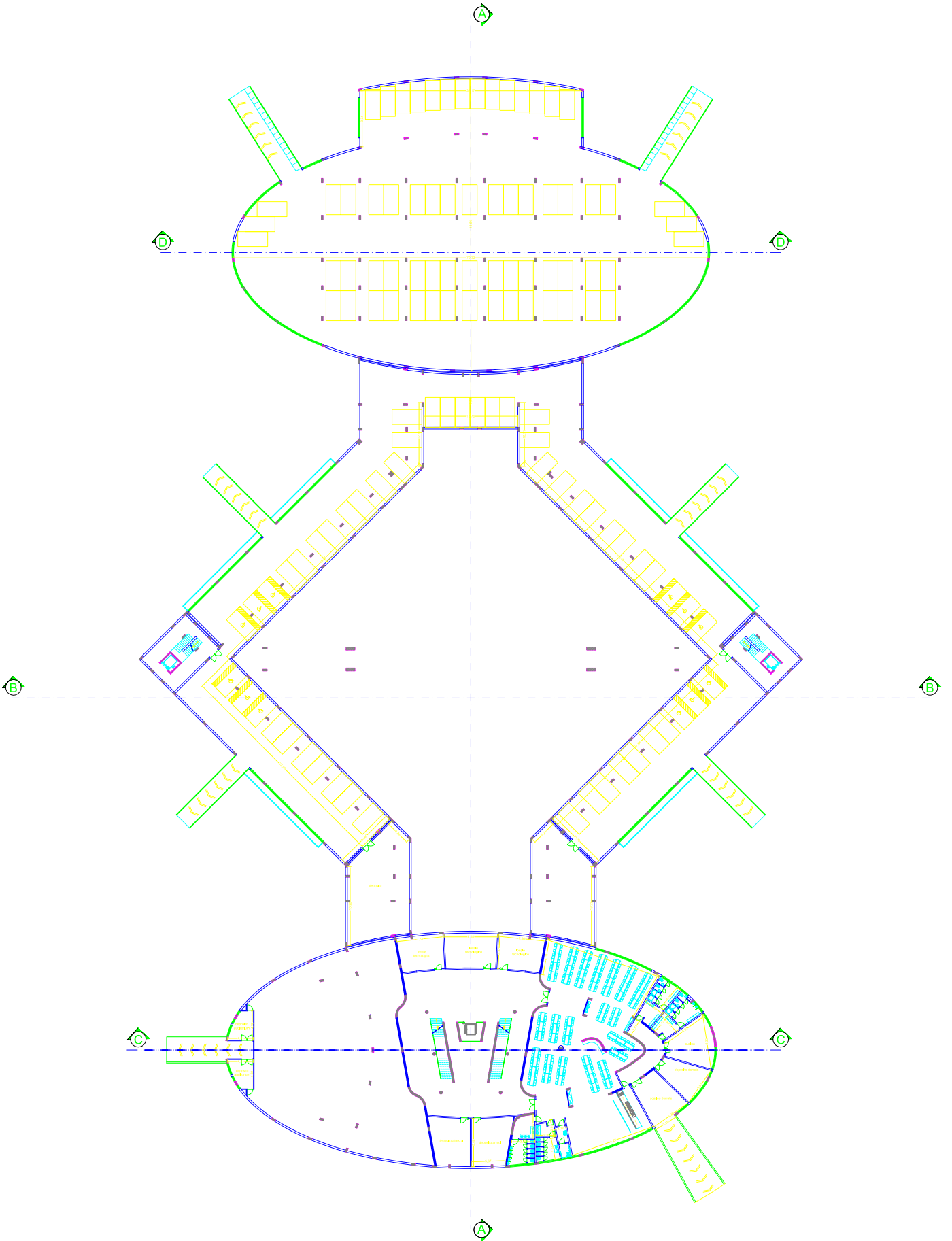
PIANTA PIANO SEMINTERRATO scala 1:200
